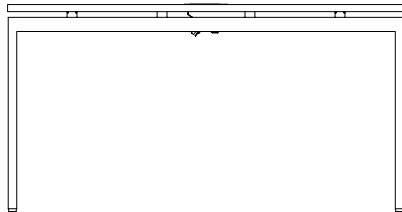
Mesa com estrutura trave
