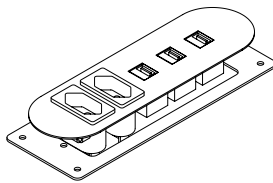
PLUGPLAY MODELO ANATRA Possível configurar tomadas, porém padrão é 02ELE e 03LOG.
