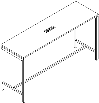
Opção com 01 Plugplay, podendo ser centralizada no tampo ou na extremidade da mesa (duto de subida e bandeja são complementos)
